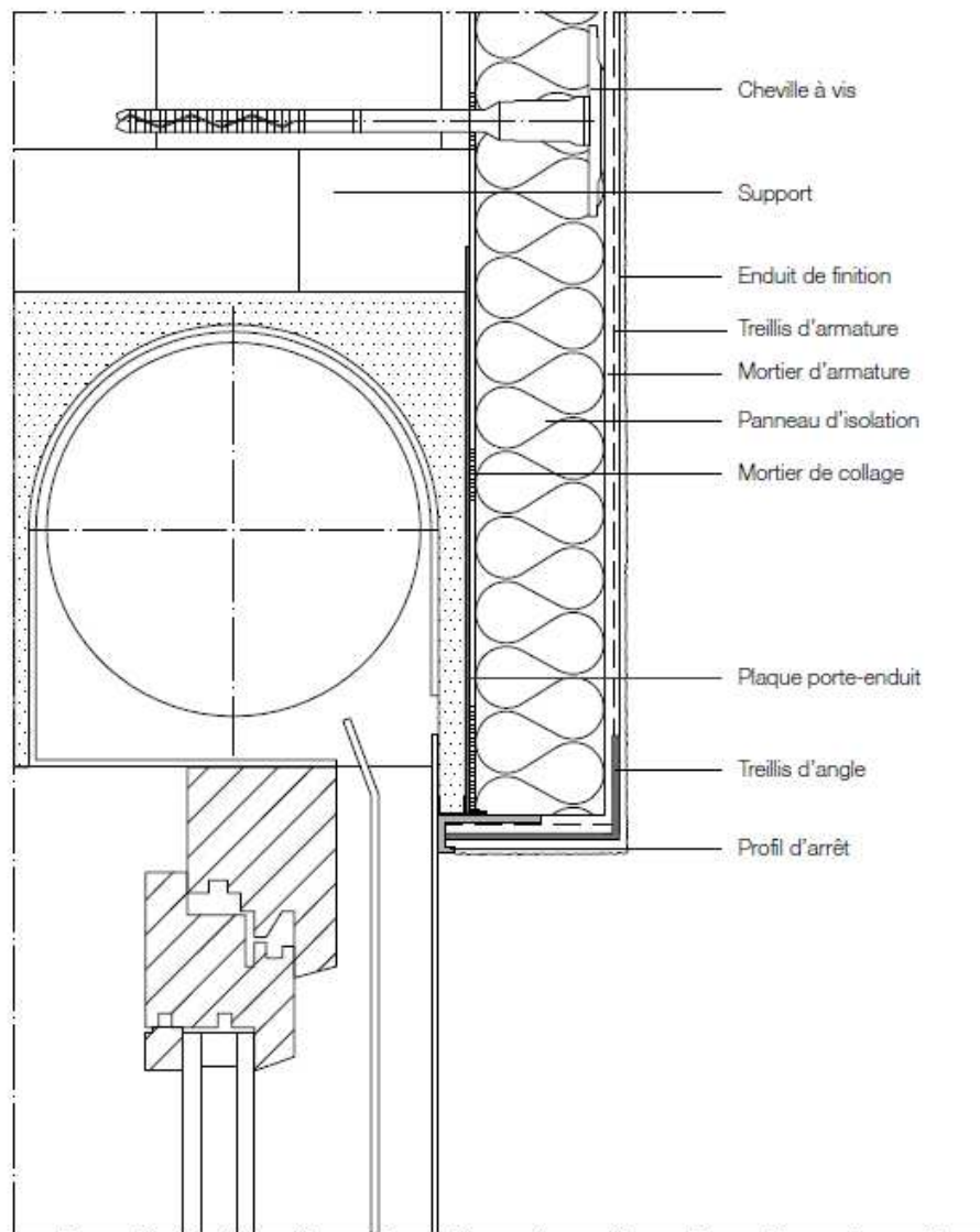
Détail coffre de volet - Sous face isolée
